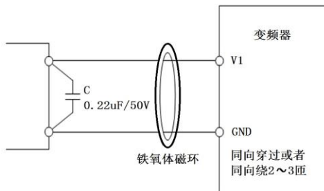
图 3-6 模拟量输入端子处理接线图
