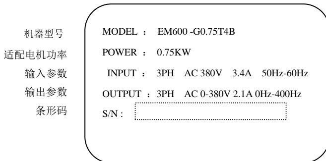
图 2-2 铭牌
