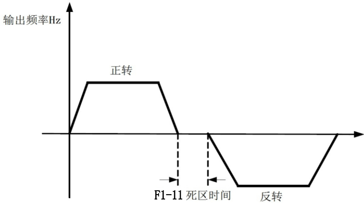
图 6-3 正反转死区时间示意图
