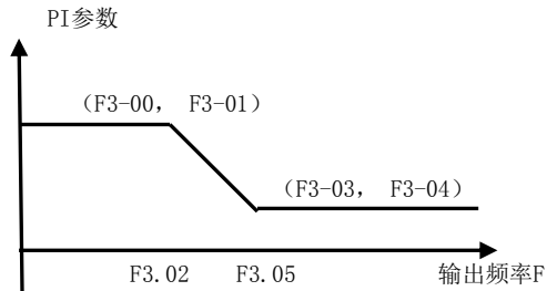
图 6-4 PI参数示意图
