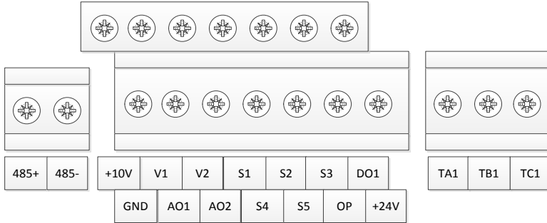
图 3-3 控制回路端子布置图
