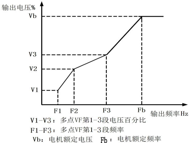
图 6-7 多点V/F曲线的设定示意图
