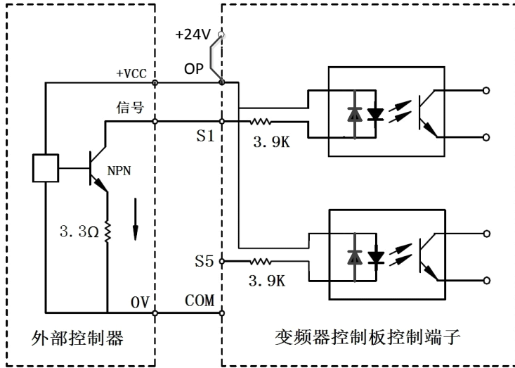
图 3-7 漏型接线方式
