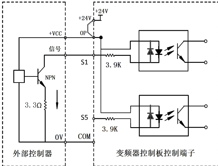
图 3-9 输入端子使用外部电源的接线方法
