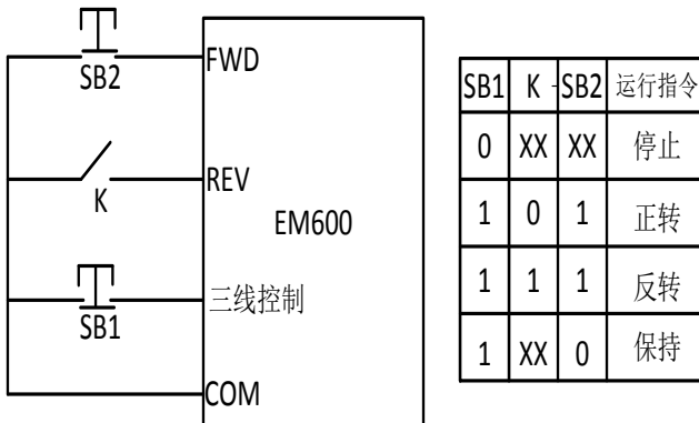
图 6-10 三线式控制1
