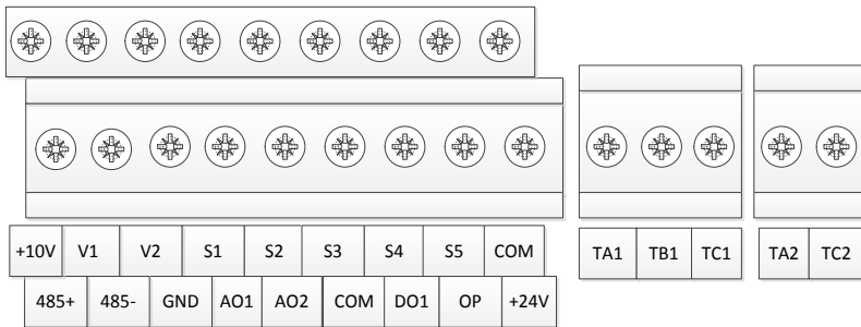
图 3-4 控制回路端子布置图
