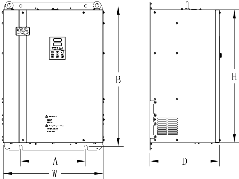
图 2-4 EM600系列金属机箱结构外型尺寸及安装尺寸示意图
