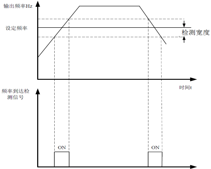
图 6-16 设定频率到达检测宽度示意图
