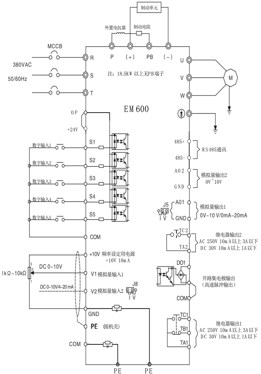
图 3-2 三相380V主回路和控制回路接线方式
