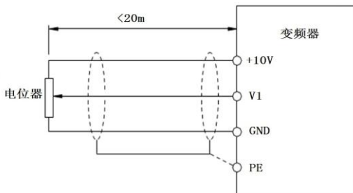
图 3-5 模拟量输入端子接线示意图
