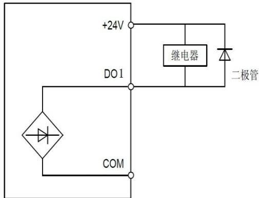
图 3-10 数字输出端子接线示意图
